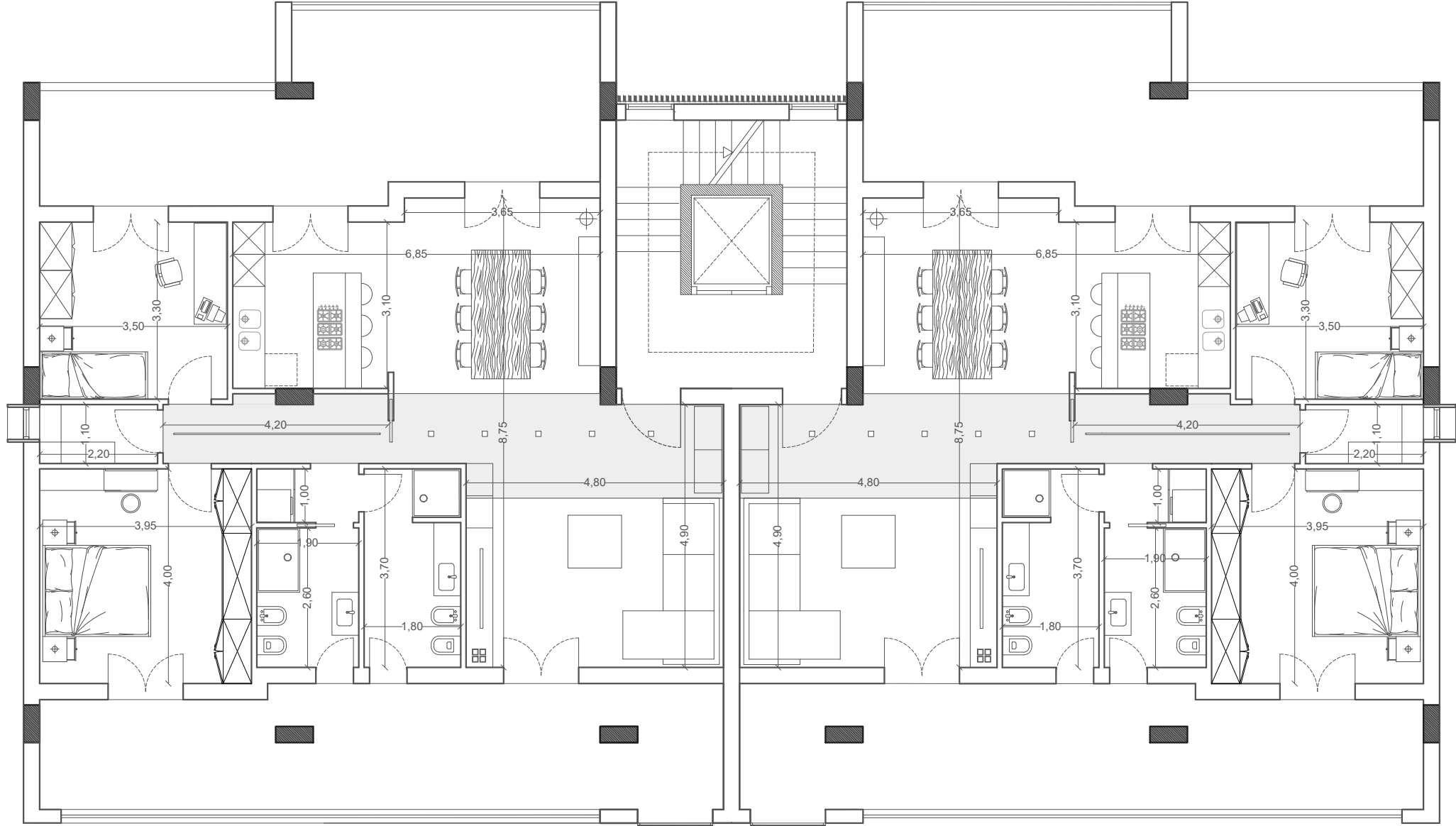
PIANTA PIANO TIPO 1:100
